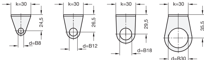
Čelní pohledy pro různé průměry otvoru - Ø d
