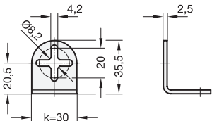
Čelní pohledy pro různé průměry otvoru - Ø d
